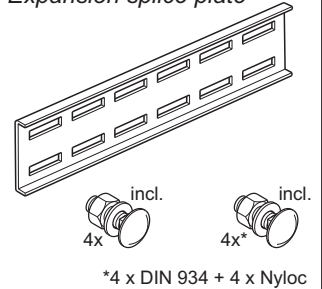
Expansie koppelplaat Expansion splice plate
