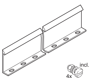
Scheidingsschot H86 Separation strip H86
