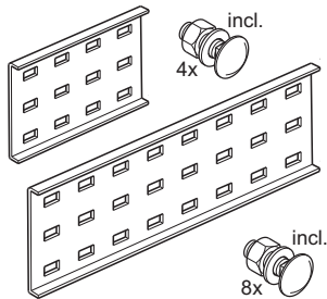
Koppelplaat 200/500 Splice plate 200/500
