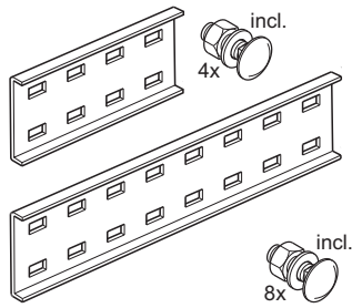
Koppelplaat 200/500 Splice plate 200/500
