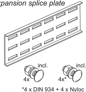
Expansie koppelplaat Expansion splice plate
