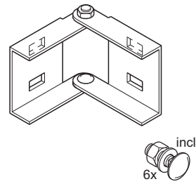
Horiz. scharn. koppelplaat Horiz. hinged splice plate
