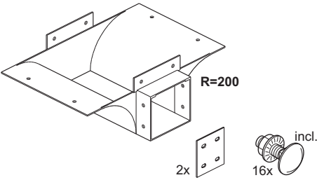
Bodemaansluitstuk Bottom connection piece
