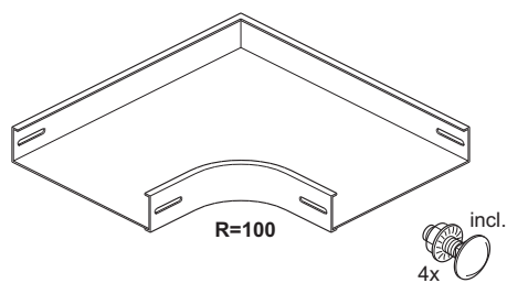
Hoekstuk 90° Corner piece 90°
