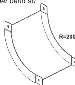
Stijgstuk 90° Vertical inner bend 90°
