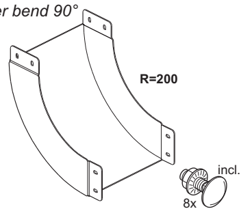
Stijgstuk 90° Vertical inner bend 90°
