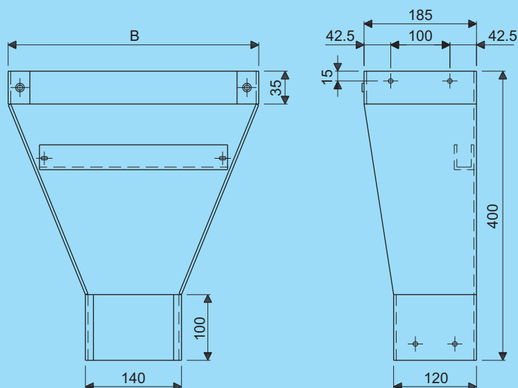
Aansluitstukdeksel voor junction box Connection piece cover for junction box
