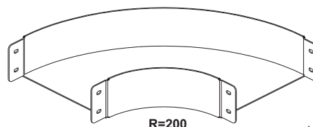
Horizontaal bochtstuk 90° Horizontal bend 90°
