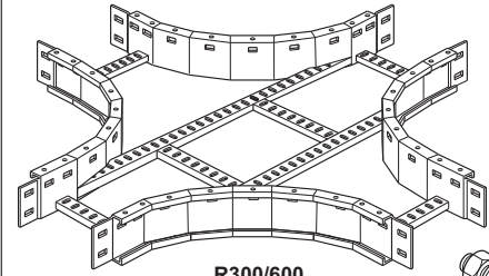
Vierwegstuk Cross piece
