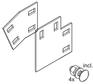
Hoekkoppelplaat Corner splice plate
