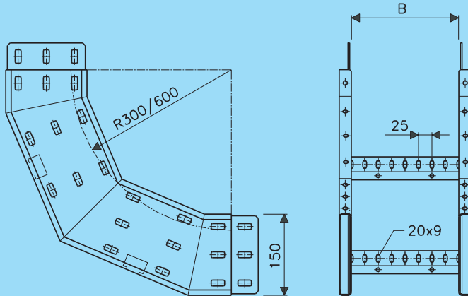
Stijgstuk 90° Vertical inner bend 90°
