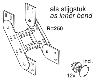
Verticaal bochtstuk 90° Vertical bend piece 90°
