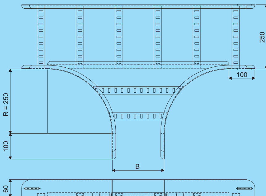
Driewegstuk Tee piece
