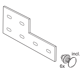
Overgangskoppelplaat Height reducing splice plate
