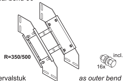
Verticaal bochtstuk 90° Vertical bend 90°
