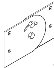
Vert. scharn. koppelplaat Vert. hinged splice plate
