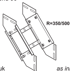
Verticaal bochtstuk 90° Vertical bend 90°
