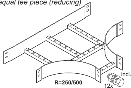
Driewegstuk (ongelijkzijdig) Unequal tee piece (reducing)
