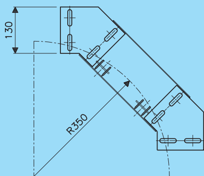
Verticaal bochtstuk 90° Vertical bend 90°
