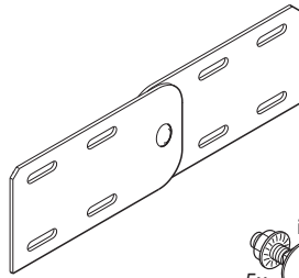
Scharnierende koppelplaat Hinged splice plate
