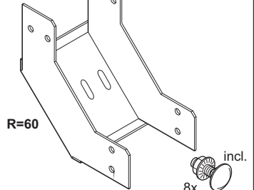
Stijgstuk 90° Vertical inner bend 90°
