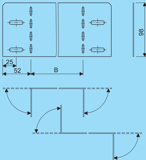
Eindschot/Verloopkoppelplaat Endplate/Reducer splice plate
