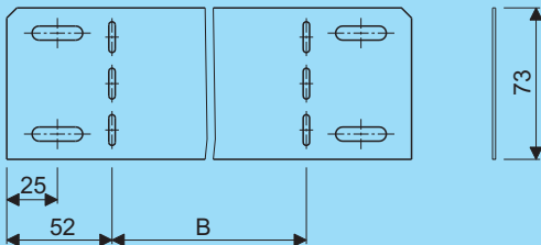
Eindschot/Verloopkoppelplaat Endplate/Reducer splice plate
