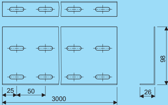
Scheidingsschot Separation strip
