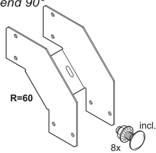
Vervalstuk 90° Vertical outer bend 90°
