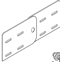
Scharnierende koppelplaat Hinged splice plate
