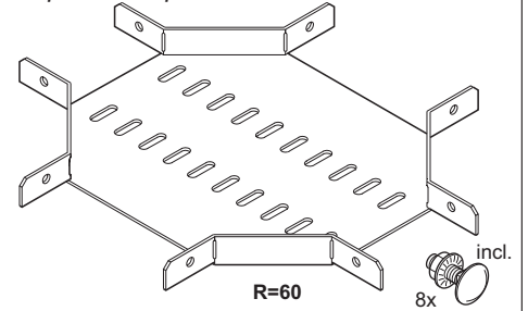
Vierwegstuk (ongelijkzijdig) Unequal cross piece
