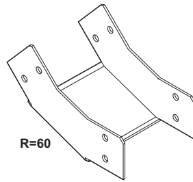
Stijgstuk 45° Vertical inner bend 45°
