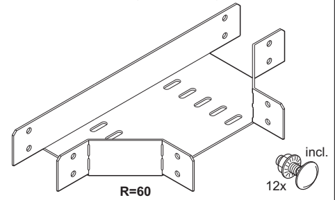
Driewegstuk (ongelijkzijdig) Unequal tee piece (expanding)
