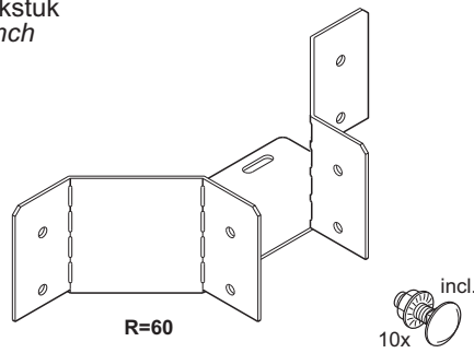
Driewegstuk (gelijkzijdig) Equal tee piece
