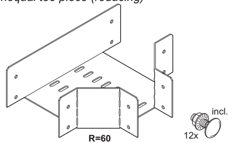
Driewegstuk (ongelijkzijdig) Unequal tee piece (reducing)
