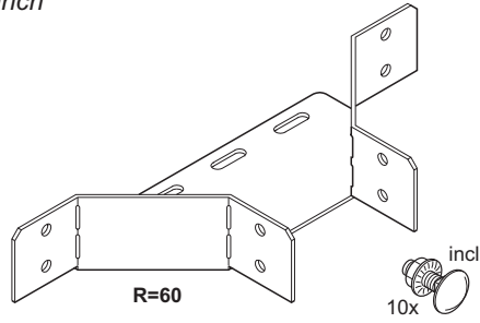
Aftakstuk Branch
