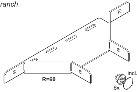
Driewegstuk (gelijkzijdig) Equal tee piece
