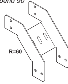
Vervalstuk 90° Vertical outer bend 90°
