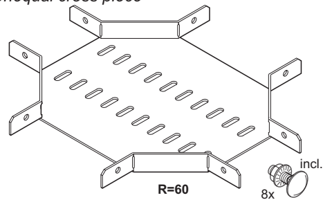
Vierwegstuk (ongelijkzijdig) Unequal cross piece
