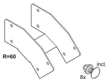
Vervalstuk 45° Vertical outer bend 45°
