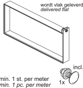
Sluitband met tape Fastener with tape
