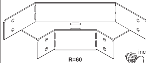
Hoekstuk 90° Corner piece 90°
