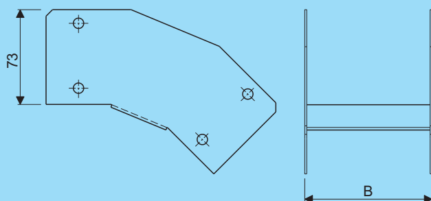
Vervalstuk 45° Vertical outer bend 45°
