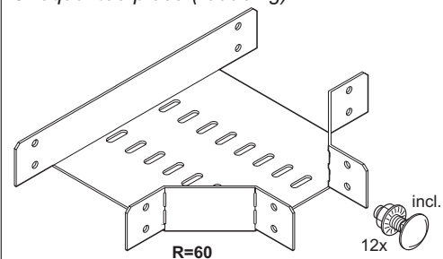
Driewegstuk (ongelijkzijdig) Unequal tee piece (reducing)
