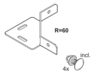
Aanzethoekstuk Universal corner piece
