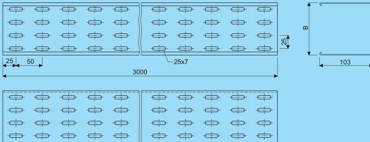
Kabelkanaal - H103R Cable duct - H103R
