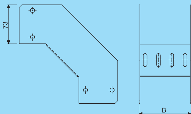
Vervalstuk 90° Vertical outer bend 90°
