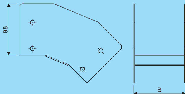
Vervalstuk 45° Vertical outer bend 45°
