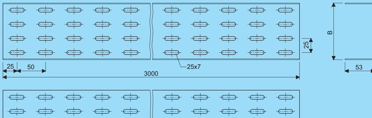
Kabelkanaal - H53 Cable duct - H53
