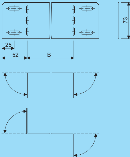
Eindschot/Verloopkoppelplaat Endplate/Reducer splice plate
