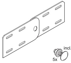
Scharnierende koppelplaat Hinged splice plate
