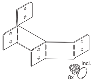
Verloopstuk Reducer
