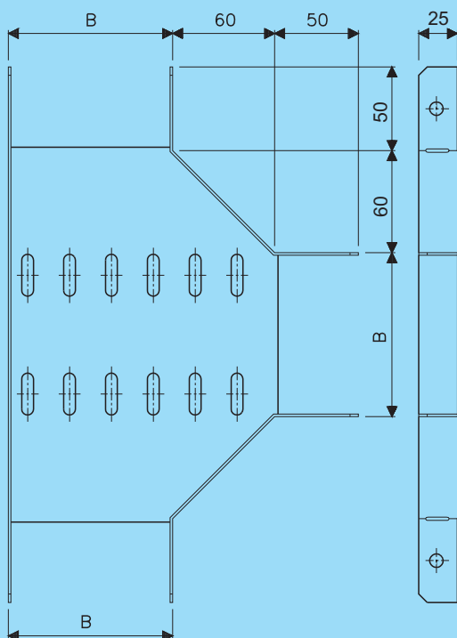
Driewegstuk (gelijkzijdig) Equal tee piece
