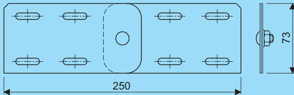
Scharnierende koppelplaat Hinged splice plate
