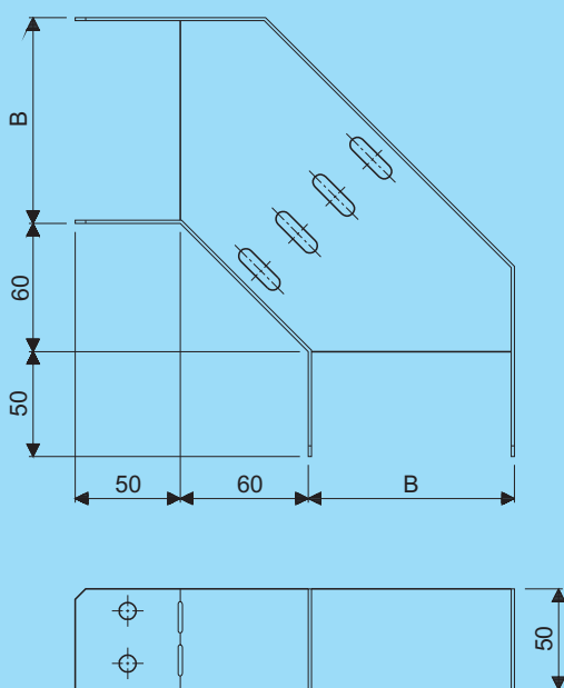
Hoekstuk 90° Corner piece 90°
