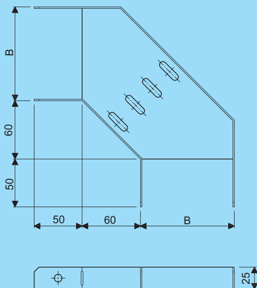
Hoekstuk 90° Corner piece 90°
