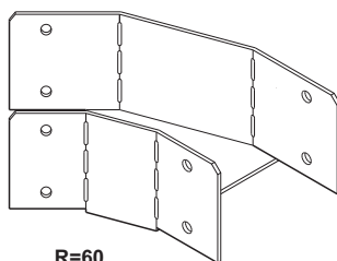
Hoekstuk 45° Corner piece 45°
