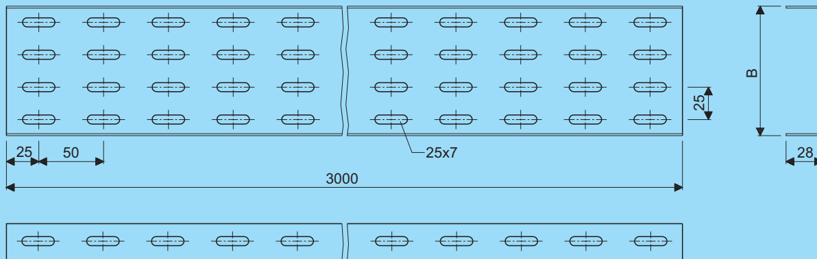
Kabelkanaal - H28 Cable duct - H28
