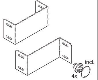
Eindschot/Verloopkoppelplaat Endplate/Reducer splice plate
