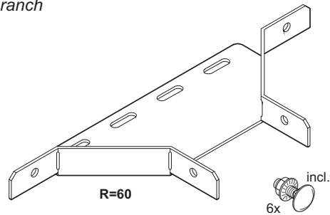
Aftakstuk Branch
