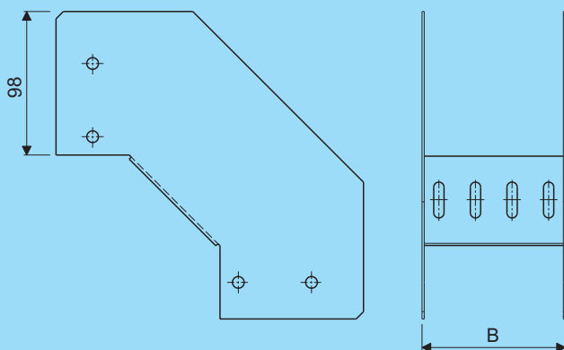
Vervalstuk 90° Vertical outer bend 90°
