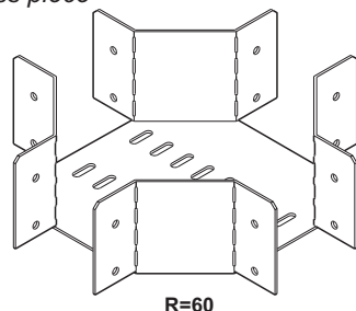
Vierwegstuk Cross piece
