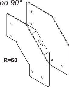
Vervalstuk 90° Vertical outer bend 90°
