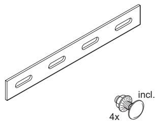
Koppelplaat Splice plate
