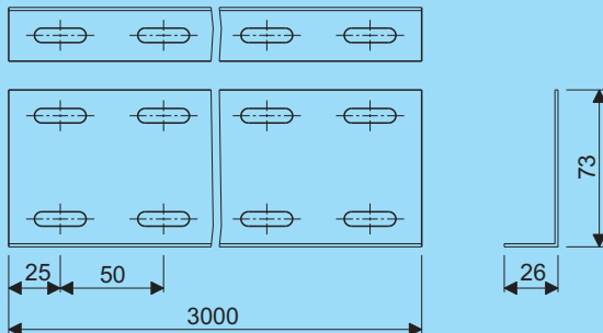
Scheidingsschot Separation strip
