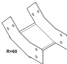
Stijgstuk 45° Vertical inner bend 45°
