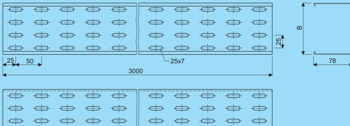
Kabelkanaal - H78R Cable duct - H78R
