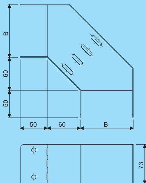
Hoekstuk 90° Corner piece 90°
